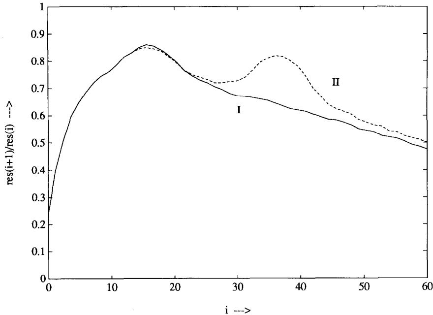
Fig. 1. GMRES; I: \alpha = 0 , II: \alpha = 0.1 .
