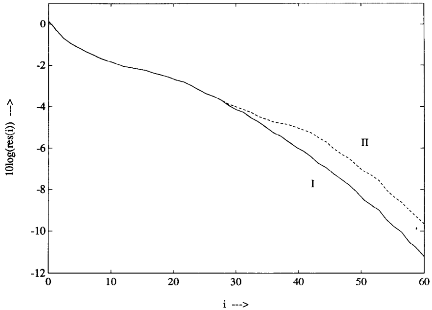
Fig. 2. GMRES; I: \alpha = 0 , II: \alpha = 0.1 .
