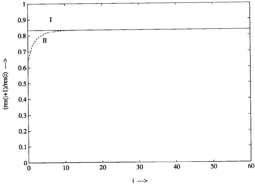
Fig. 5. \alpha = 1.2 ; I: FOM, II: GMRES.
